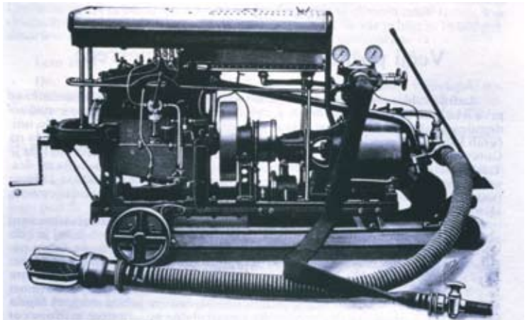
Motorna brizgalna Rosenbauer, tip Mojstrana - 1912
